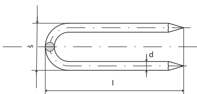
U-klince - svorky
